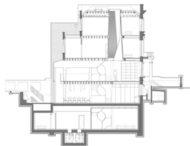
A sinistra, la sezione longitudinale evidenzia il camino di luce e gli spazi principali sovrapposti, con il soggiorno a due livelli, la biblioteca e la sala da pranzo. Sopra, la spirale del vano scale; sotto, lo spazio cucina, con la scala che scende alla media room.
